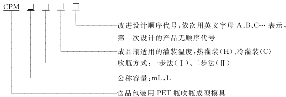
图 1 吹瓶模具的型号编制
